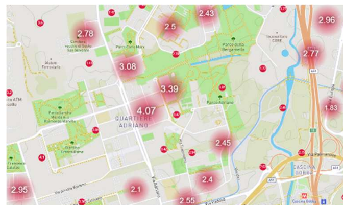
Isole di calore – dato 30 mt
